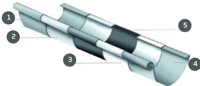
1-Acél, 2-Horganyréteg, 3-Alapozó réteg, 4-Passziváló réteg, 5-Prelaq NOVA
