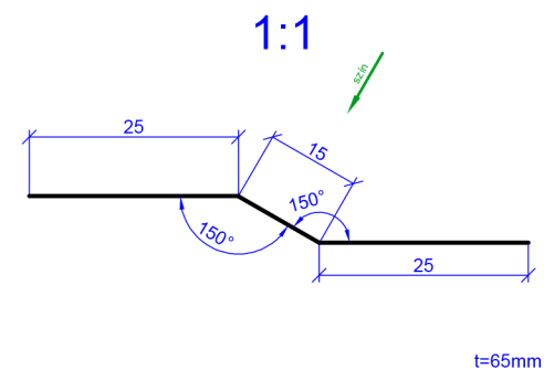
átfedő-illesztő elem
