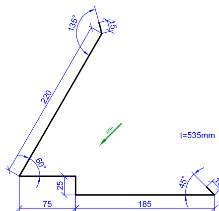
kéményszegély C
