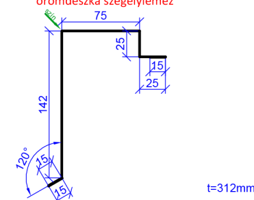
oromdeszka szegélylemez
