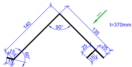
félgerinc
