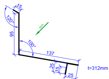
kéményszegély C
