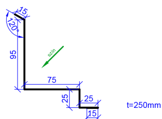
kéményszegély B
