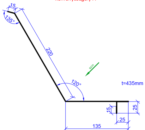
kéményszegély A
