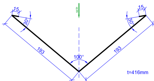
kéményszegély A
