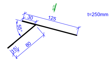
oromdeszka szegélylemez
