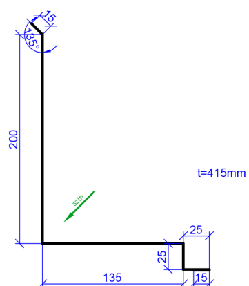
kéményszegély B
